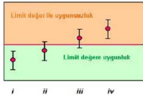
Şekil 1. Geniştirilmiş Belirsizliğin Hesaba Katıldığı Ölçüm Sonuçları İle Üst Limitin İlişkisi
