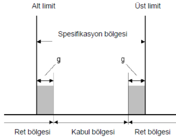
Şekil 4. Spesifikasyonda Belirtilen Üst ve Alt Limitler ve Yüksek Güvenirlik İle Kabul Kararı Alınmasını Sağlayan Bir Karar Kuralı İle Belirlenmiş Koruma Bantları, g, Karar Limitleri, Bir Kabul Bölgesi ve İki Ret Bölgesi
